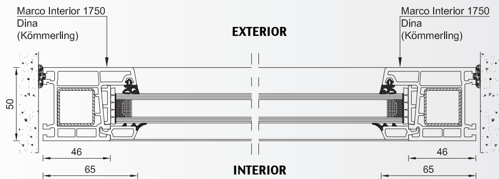
Corte B-B
