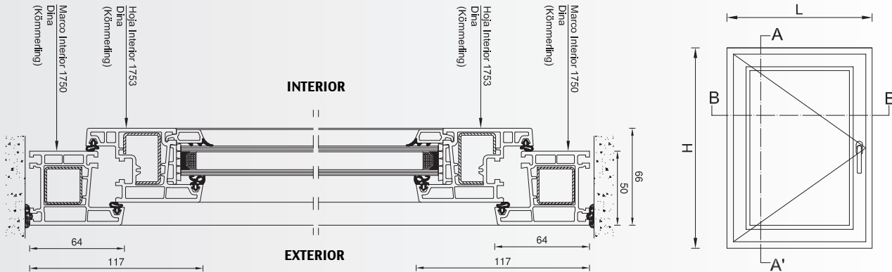
Corte A-A
