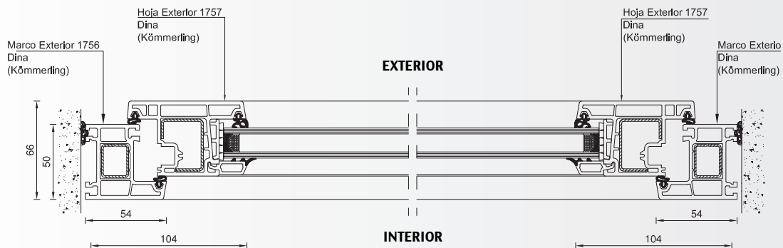
Corte B-B
