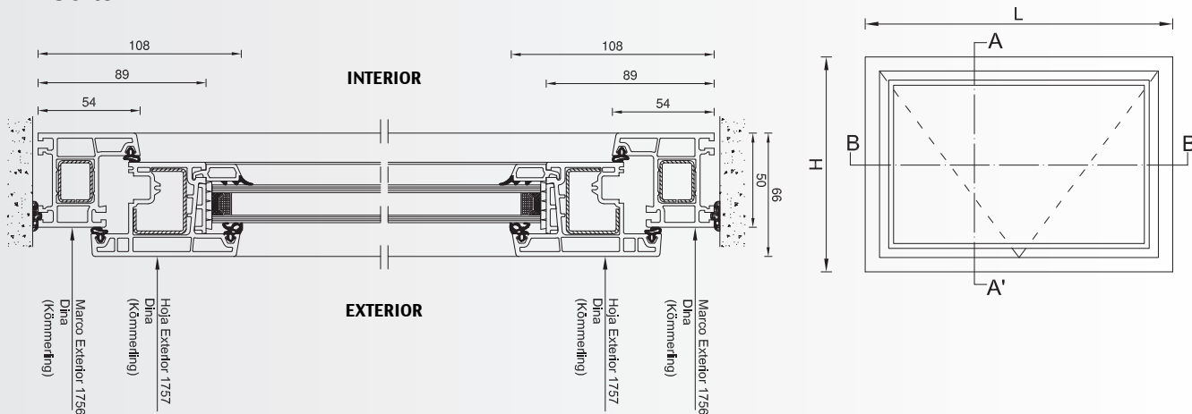
Corte A-A
